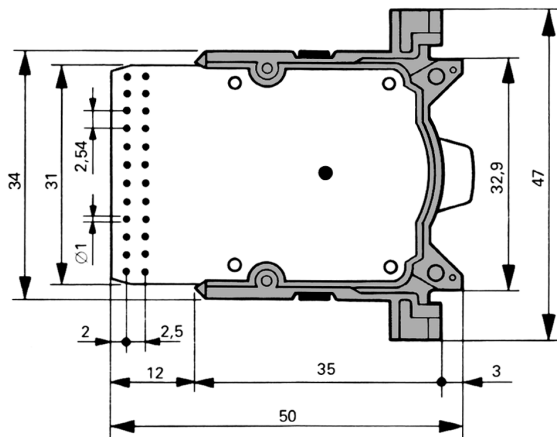
Seitenansicht
