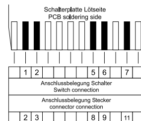
Code 531 BCD + Komplement
