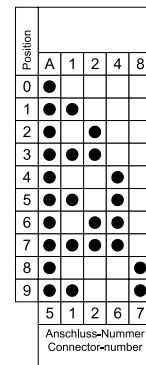
Code 044 BCD positiv kurzschliessend
